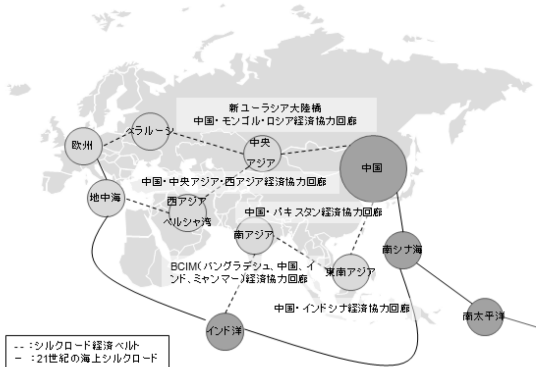
図 71 シルクロード経済ベルトと 21 世紀の海上シルクロード
